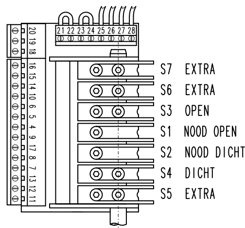
Fig. 2: Printplaat
